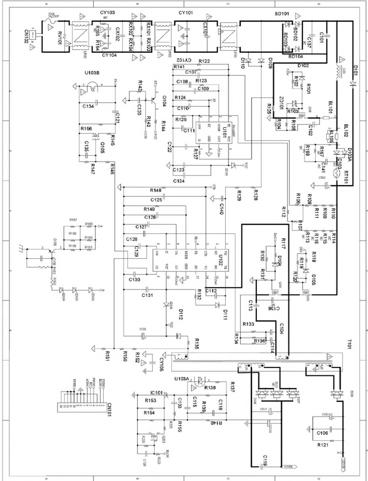
AC-DC 部分
