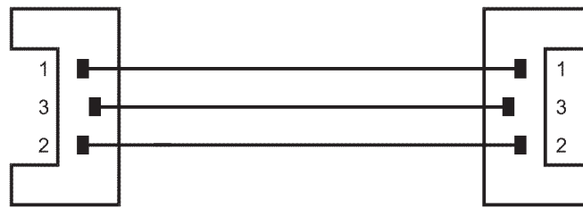
Рисунок Е.2 — Схема соединений кабеля шины
