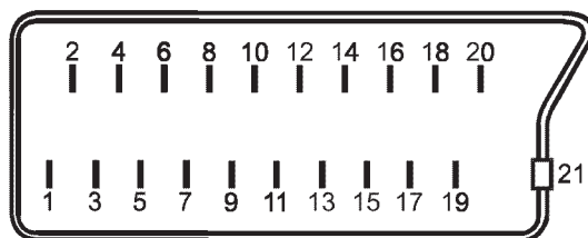
Рисунок В.1 — Расположение и нумерация контактов соединителя
