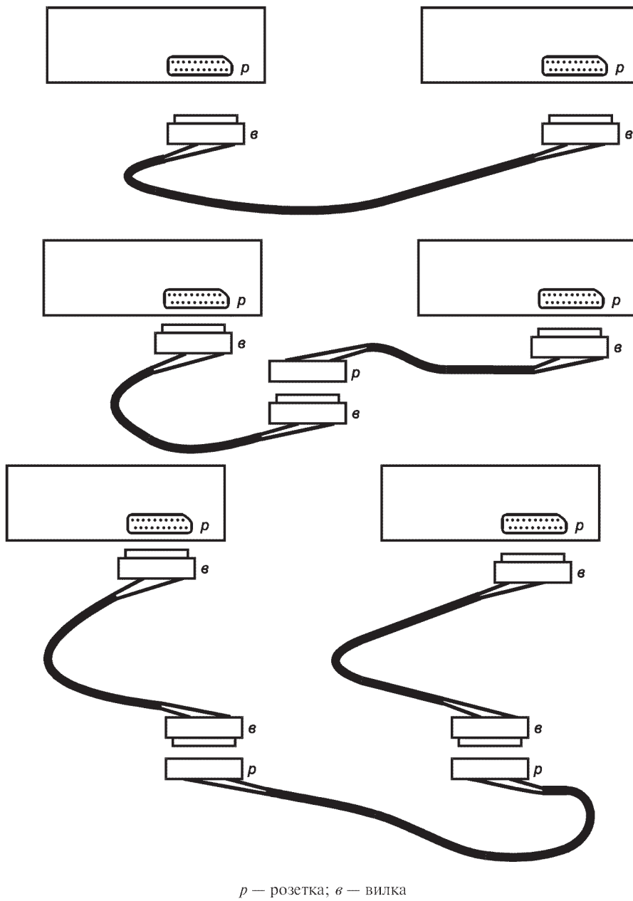
Рисунок В.2 — Виды соединительных шнуров
