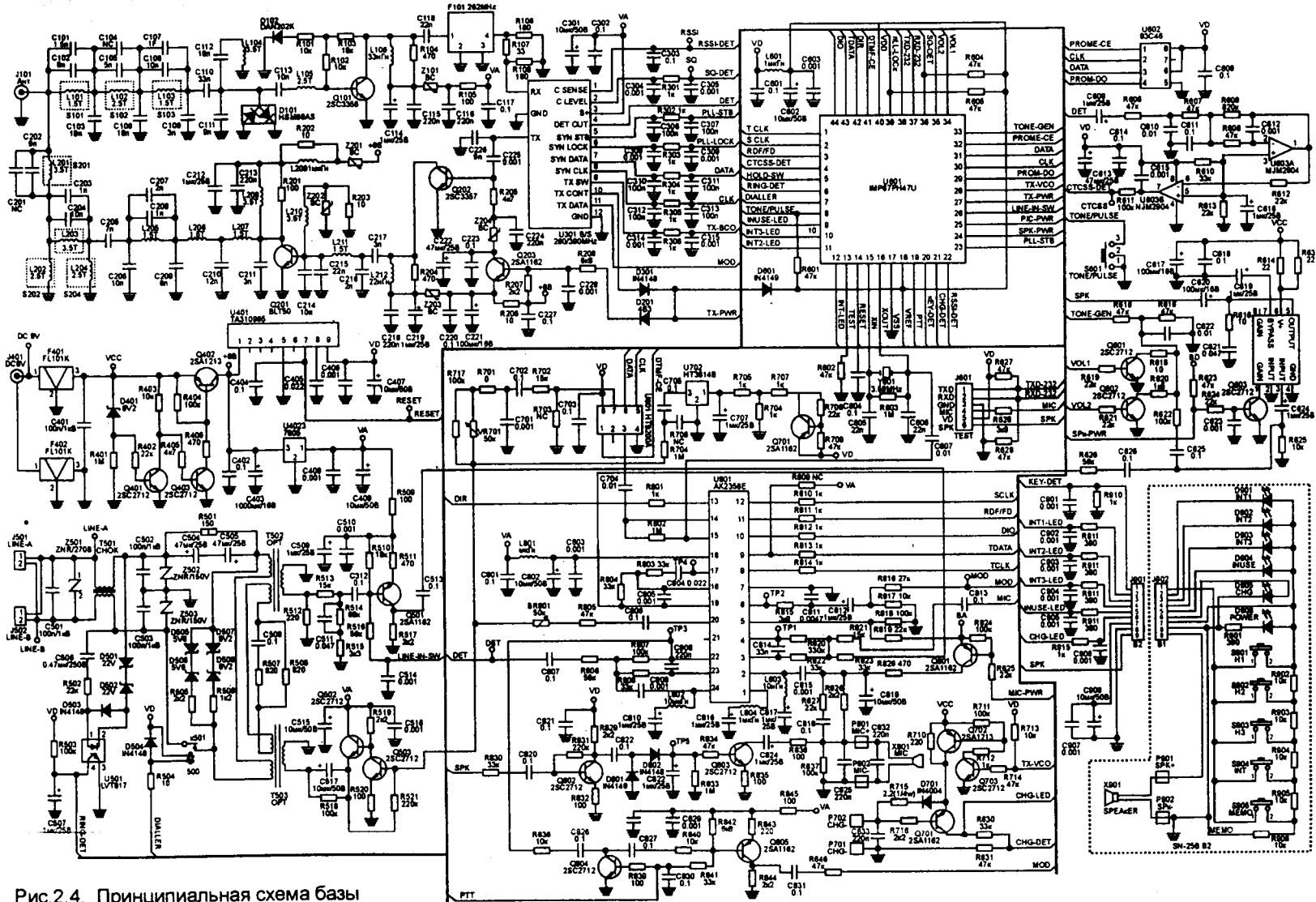
Рис.2.4. Принципиальная схема базы
