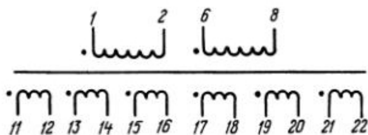
Рис2. Электрическая принципиальная схема анодного трансформатора ТА249-220-50
