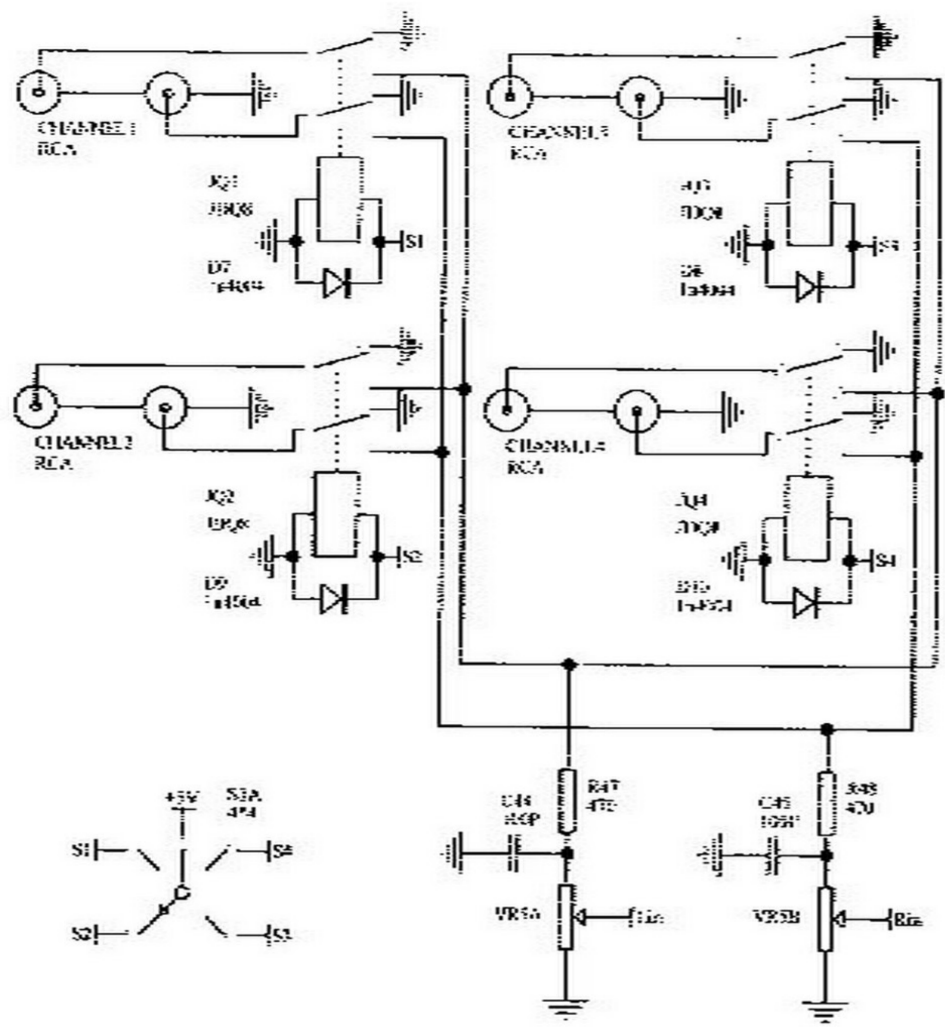
LS-100原理图 广东丽特电子公司
